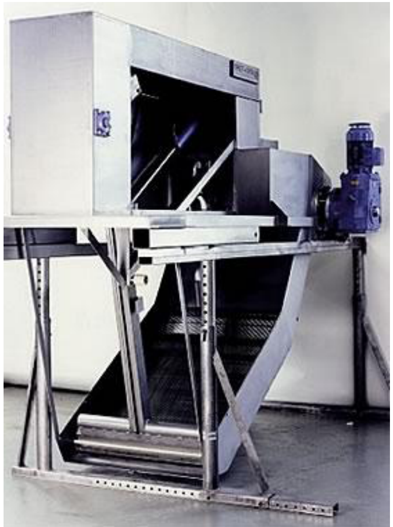
Česle typ 2.0 (díleňská fotografie): šířka kanálu = 1,0m, 400 l/s, 6 mm šířka průlin
